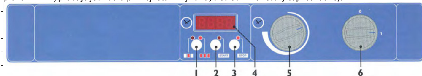
Obr. 1: Nastavení jednotky. 1 - digitální displej, 2 - tlačítko zapnutí jednotky, 3 - tlačítko start, 4 - tlačítko stop, 5 - regulace teploty, 6 - regulace výkonu.
